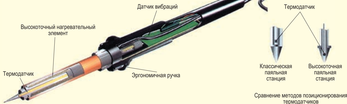
Рисунок 4 Конструкция паяльника станций серии 203 и 204
