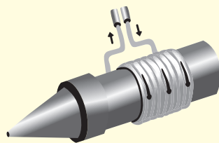
Рисунок 3 Возбуждающая обмотка паяльника станций 203 и 204
