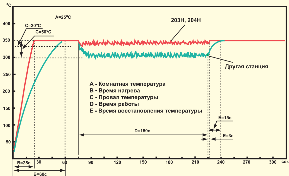
Рисунок 5 Графики температурных характеристик индукционных и классических паяльных станций
